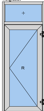
Enkeldörr med överljus Helglasad
