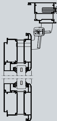
Fritt öppningsmått 90 grader enkeldörr: Karmyttermått -212 B-B
