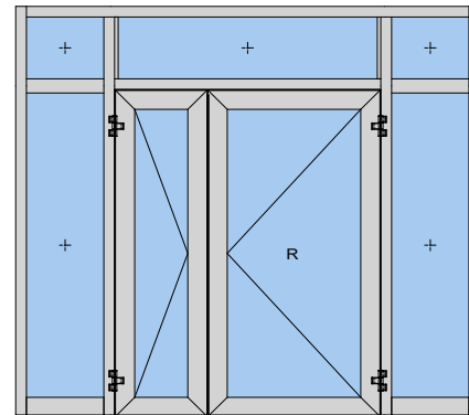
Pardörr med sido- och överljus Helglasad
