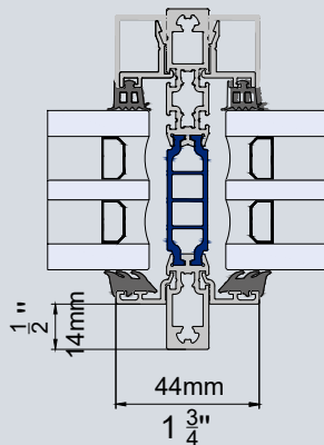
Utvändig glasning
