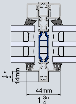
Invändig glasning
