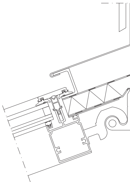
Anslutning mot vägg i överkant glastak
