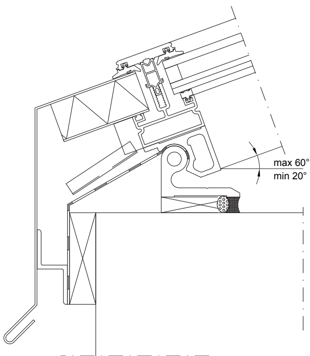
Avslutning i nederkant glastak mot sarg
