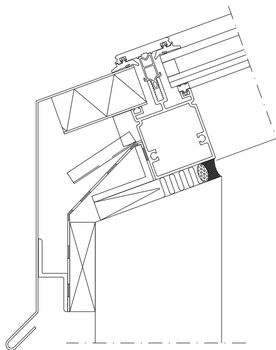
Avslutning i nederkant glastak mot sarg
