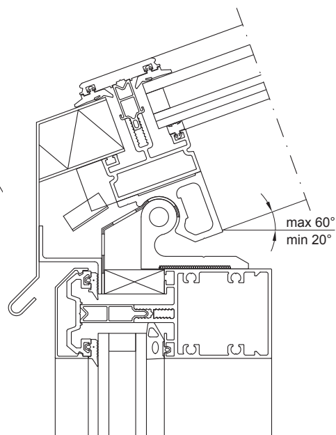
Glastak övergång till fasad 4150
