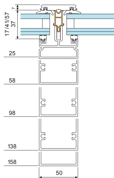
Stomprofil horisontalt enkelglas
