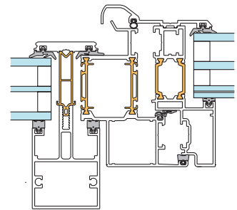
Lucka, 2- eller 3-glas isolerruta
