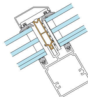
3-glas i alternativ med horisontella dekorprofiler 45° alt. 60° fasning
