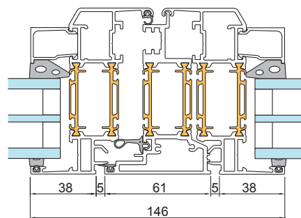
6 - Mötesfönster båge/båge 1086
