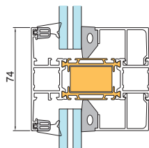
Spröjsprofil
