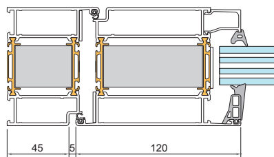
Karm/dörrblad modulprofil
