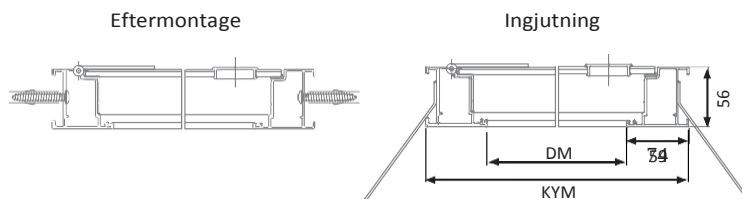
VikingShield™ 20 nedfälld lucka
