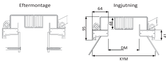
VikingShield™ 10 överfalsad isolerad lucka
