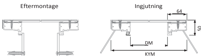
VikingShield™ 30 nedfälld tät lucka
